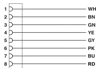
Kontaktbelegung der M12-Buchse
