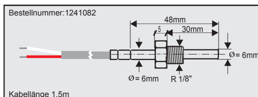
Flüssigprobe - St-St-Gehäuse
