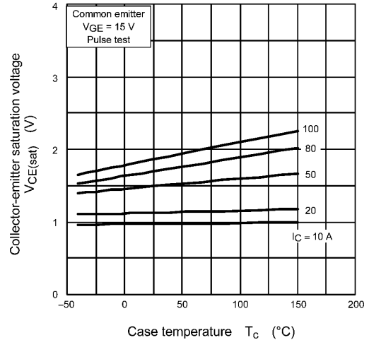
Fig. 8.4 V_{CE(sat)} - T_c
