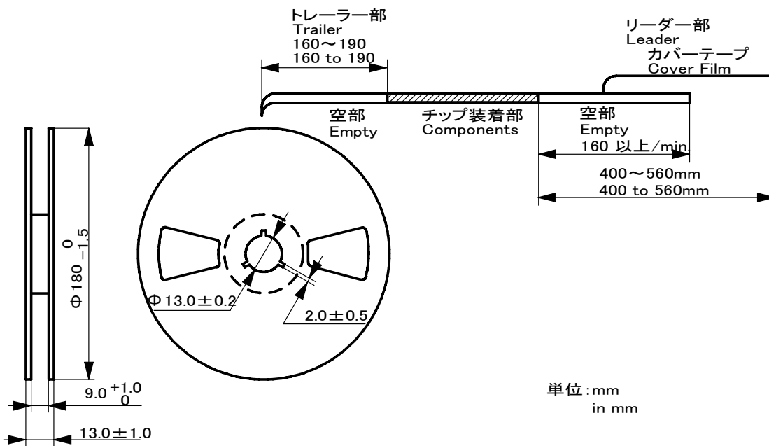
第4図 プラスチックリールの外形寸法図 Figure 4. Dimensions of Plastic Reel (CSTCE16M0V53A-R0)
