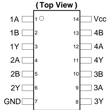
SO-14 / TSSOP-14
