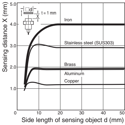
E2A-S08□N04/M08□N04
