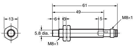
E2A-S08LN04-M5-□□
