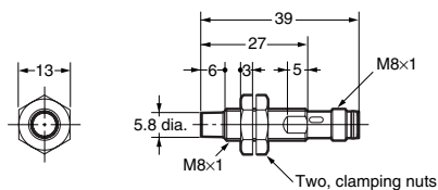
E2A-S08KN04-M5-□□
