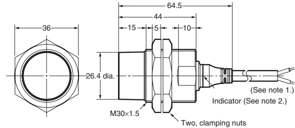
E2A-M30KN20-WP-□□
