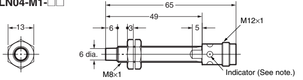
E2A-S08LN04-M1-□□ E2A-M08LN04-M1-□□
