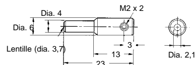
E39-F3A Lentille de l'unité de réflexion
