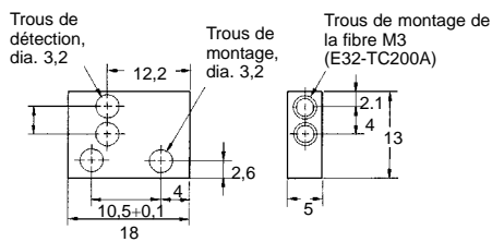
E39-F5 Kit de conversion pour réflexion diffuse latérale
