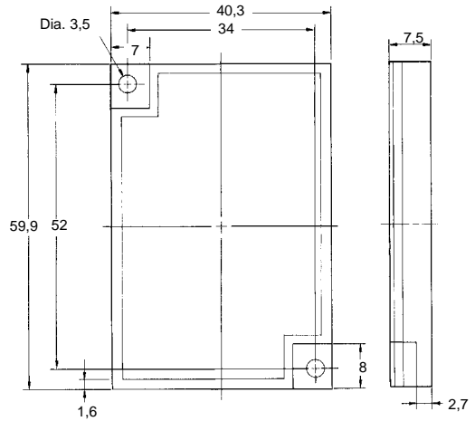
Réflecteur (bande) E39-RSB (à commander séparément)
