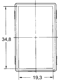
Réflecteur (bande) E39-RSA (à commander séparément)
