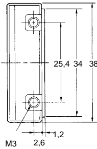
Réflecteur (bande) E39-RSA (à commander séparément)
