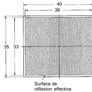
Réflecteur (bande) E39-RSB (à commander séparément)
